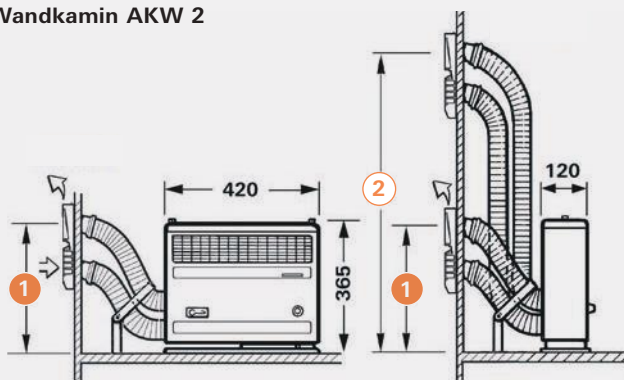
Einbauvarianten
